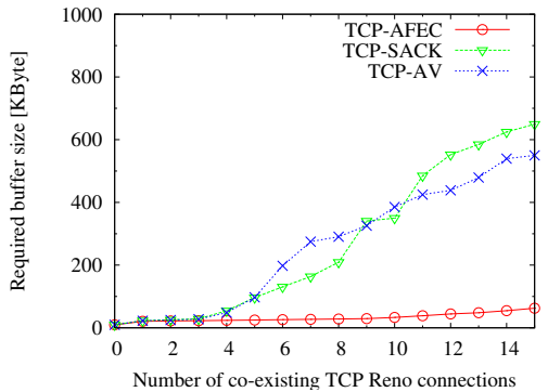
図 9 受信ホストに必要なバッファサイズの変化 (95%分位点) .
