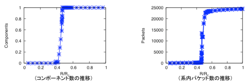
BA AT&Tポロジでのシミュレーション結果
